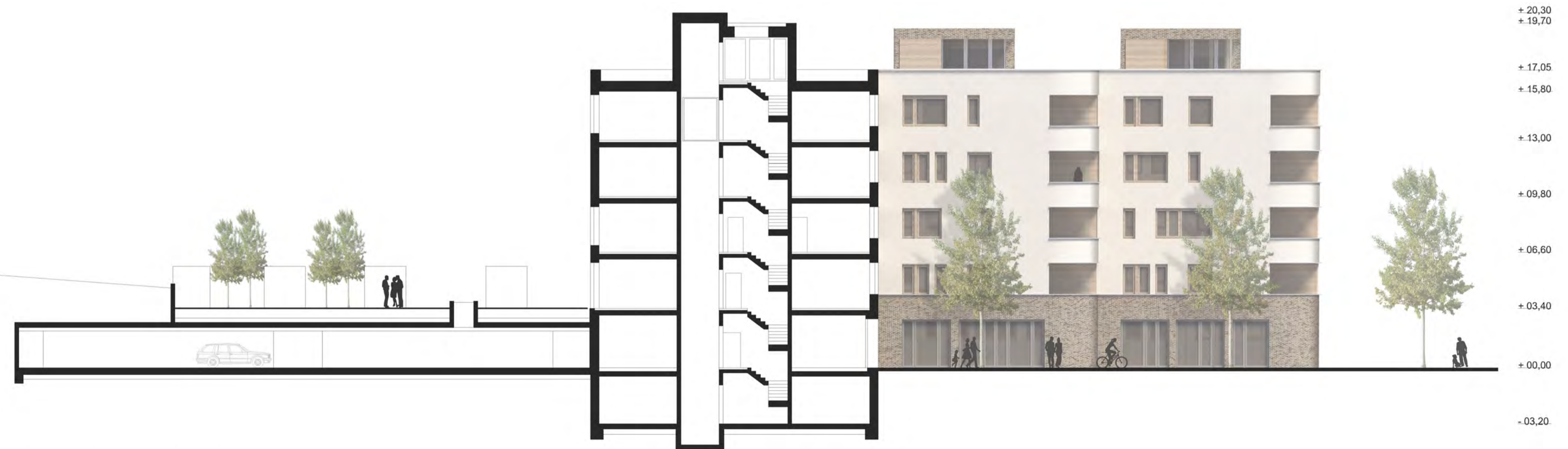
SCHNITT CC M 1.200
